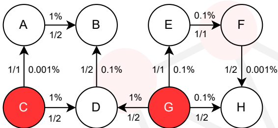
Figura 1: Red social inicial. Los NM están resaltados en rojo.
