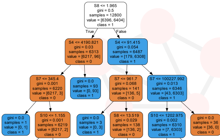
Figura 4: Árbol de decisión.
